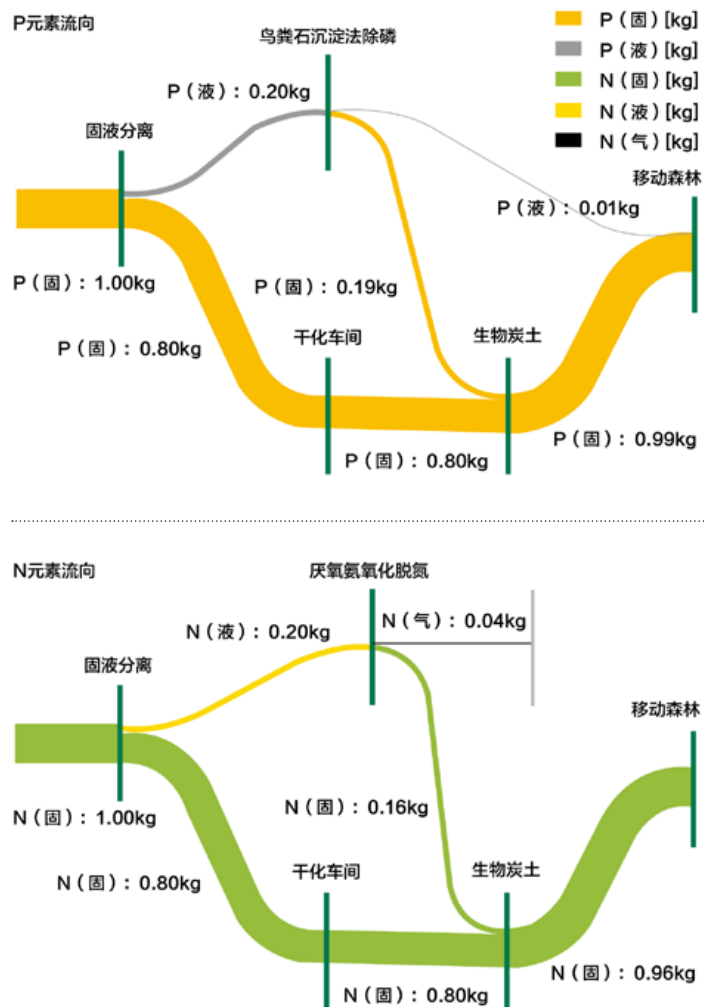
图 5 | 鱼梁洲项目氮、磷平衡示意图
