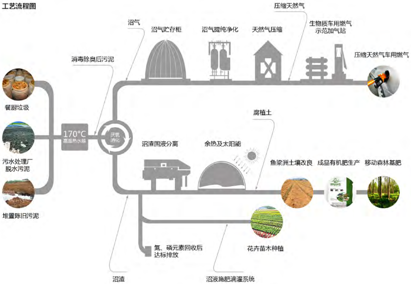
图 3 | 鱼梁洲项目流程图
