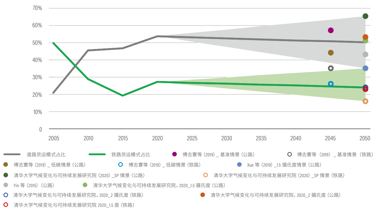
图 13 | 现有文献对货运运输结构(周转量占比)的预测
