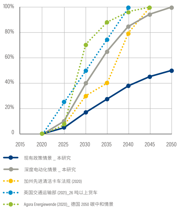
a. 新能源中重型货车的市场渗透率
