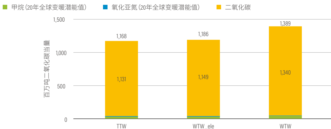
图 24 | 2020年不同核算范围下的道路交通温室气体排放量
