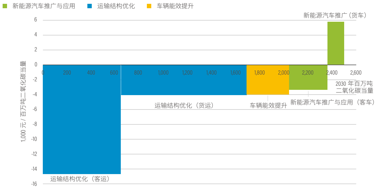
图 40 | 边际减排成本曲线:2030年
