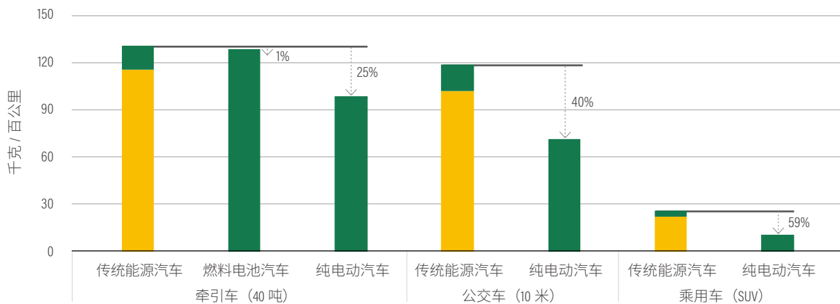
图 21 | 当前发电结构（2020年）和氢气供给结构（2018年）下各车型“油井到车轮”二氧化碳排放量
