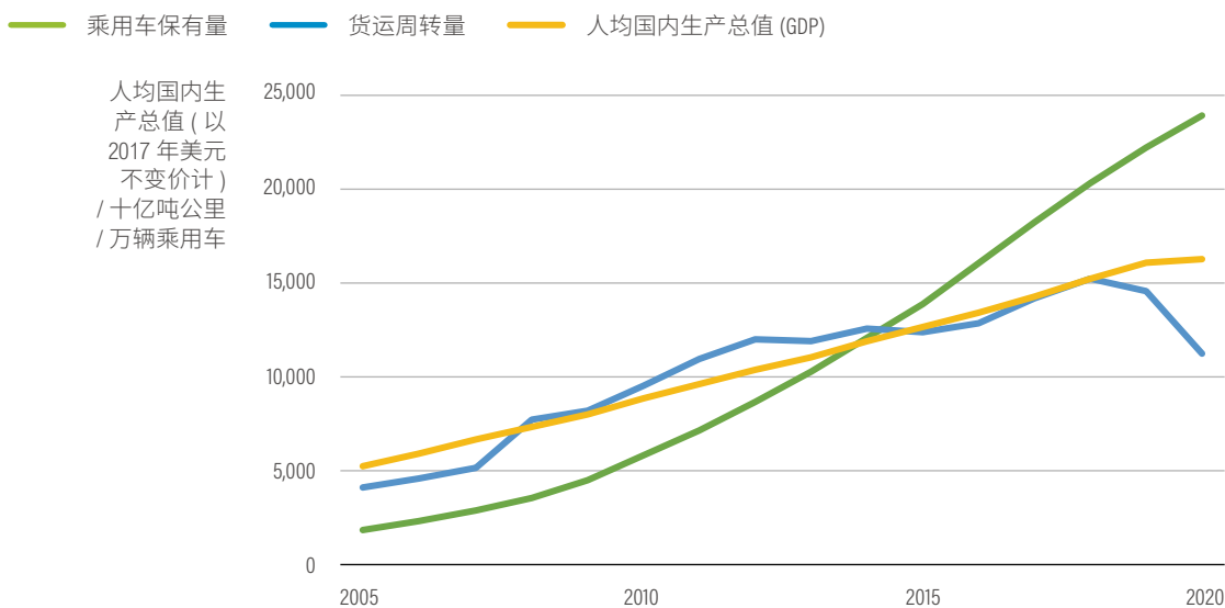
图 5 | 2005年至2020年乘用车保有量、货运周转量和人均国内生产总值的增长情况
