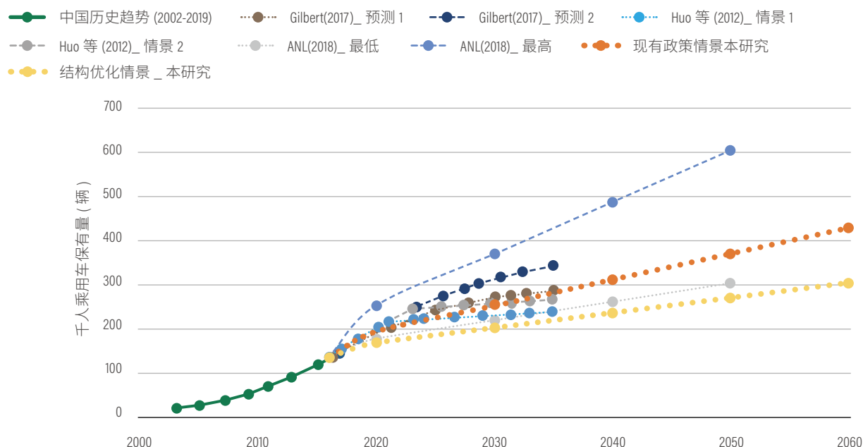
图 7 | 本研究与各文献对国内未来千人乘用车保有量的预测
