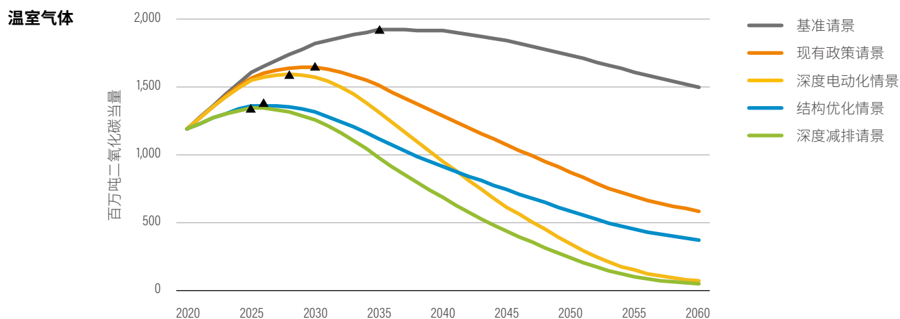
图 26 | 不同情景下的二氧化碳与温室气体排放
