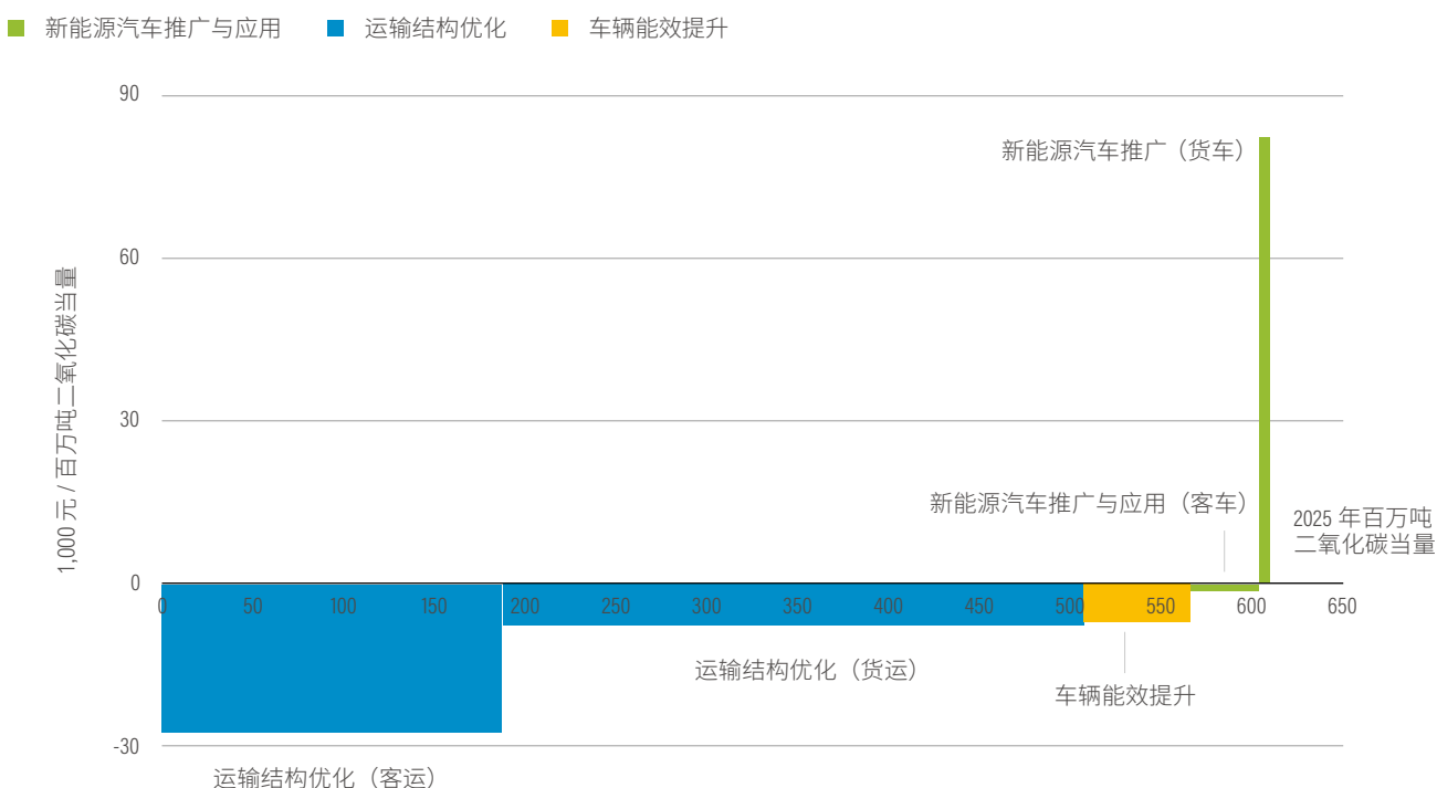
图 39 | 边际减排成本曲线:2025年
