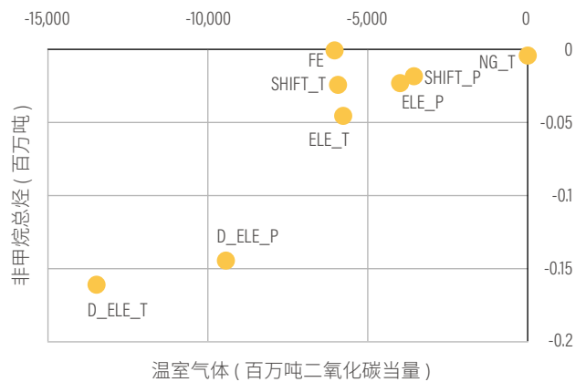
非甲烷总烃和温室气体的协同效应(2035—2060年)
