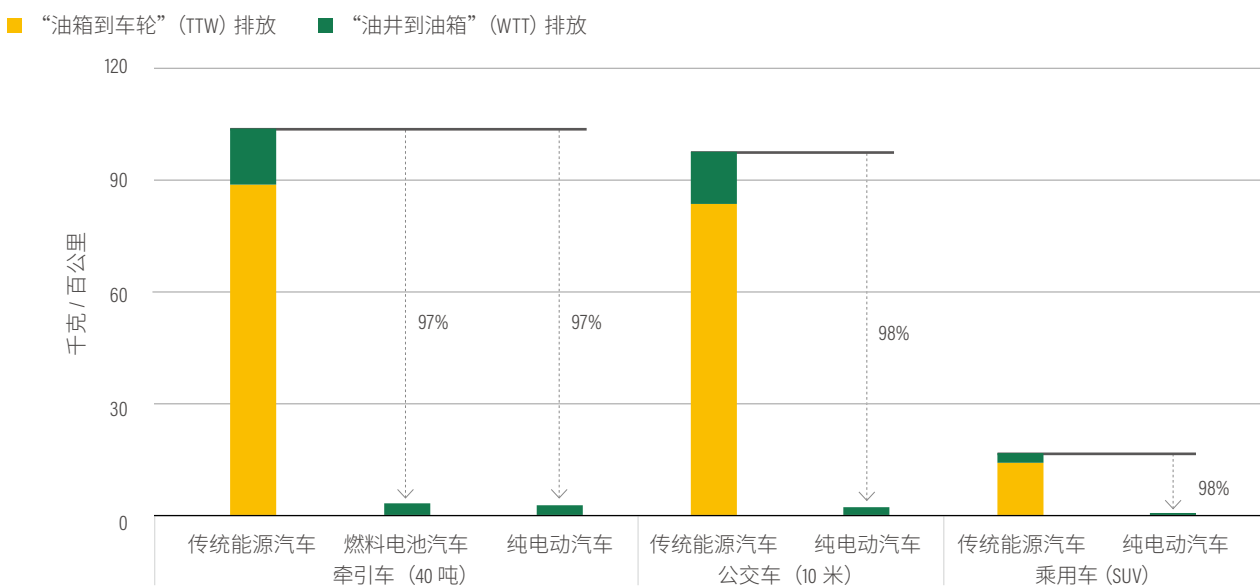
图 23 | 现有政策情景2050年的发电结构和氢气供给结构下各车型“油井到车轮”二氧化碳排放量
