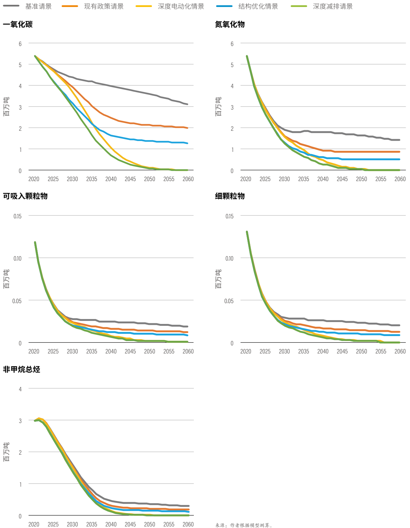
图 31 | 不同情景下道路交通空气污染物排放
