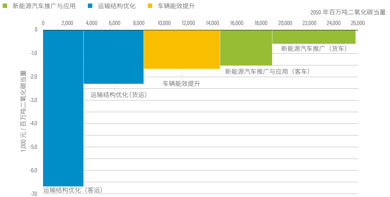
图 41 | 边际减排成本曲线:2050年
