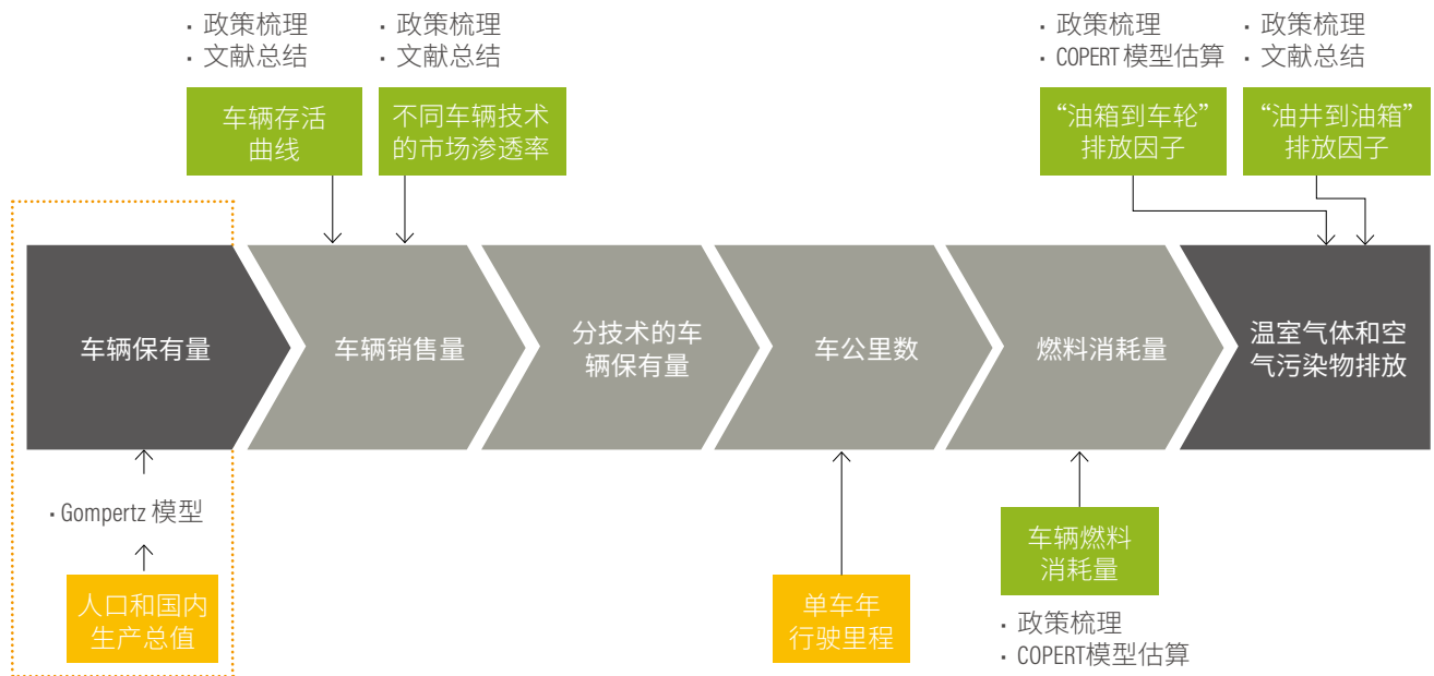
图 4 | 客运排放预测方法
