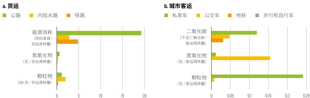
图 9 | 不同交通运输模式的能源消耗强度或碳排放强度
