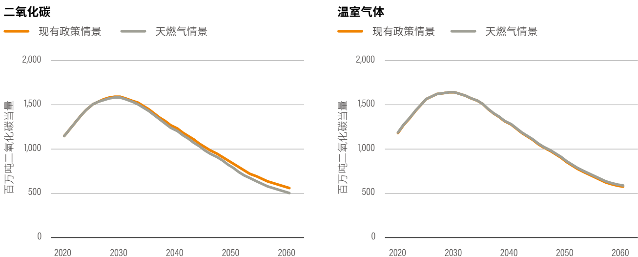
图 37 | 现有政策情景和天然气情景中二氧化碳和温室气体排放对比
