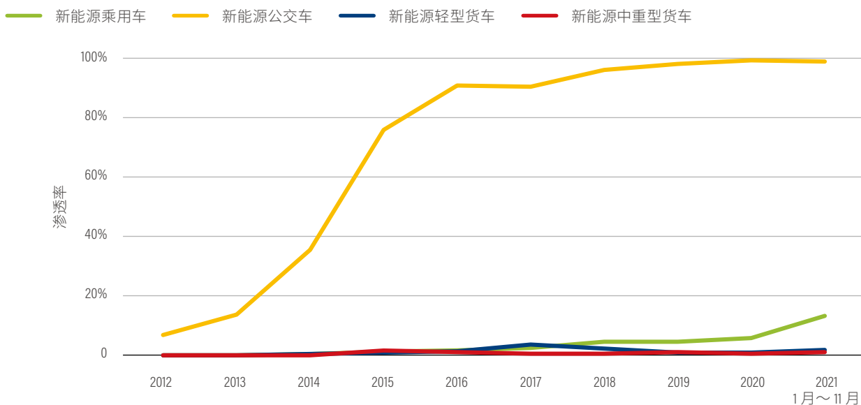
图 15 | 各类车型的新能源汽车市场渗透率(2012年—2021年11月)
