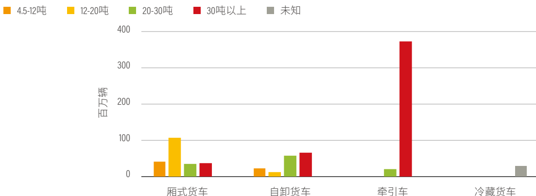
图 16 | 根据车辆总设计质量与车型划分的中重型货保有量
